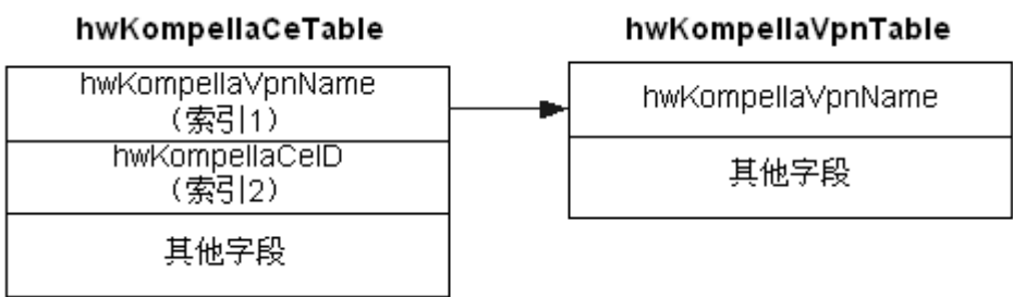
图 66-2 Kompella 方式 VPN CE 配置表和 Kompella 方式 VPN 配置表之间关系
